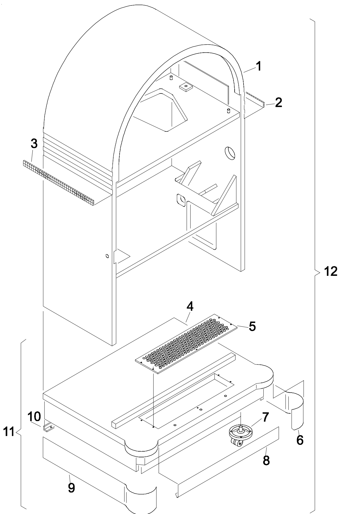
Fig. 7 - Gehäuse / Cabinet / Meuble
