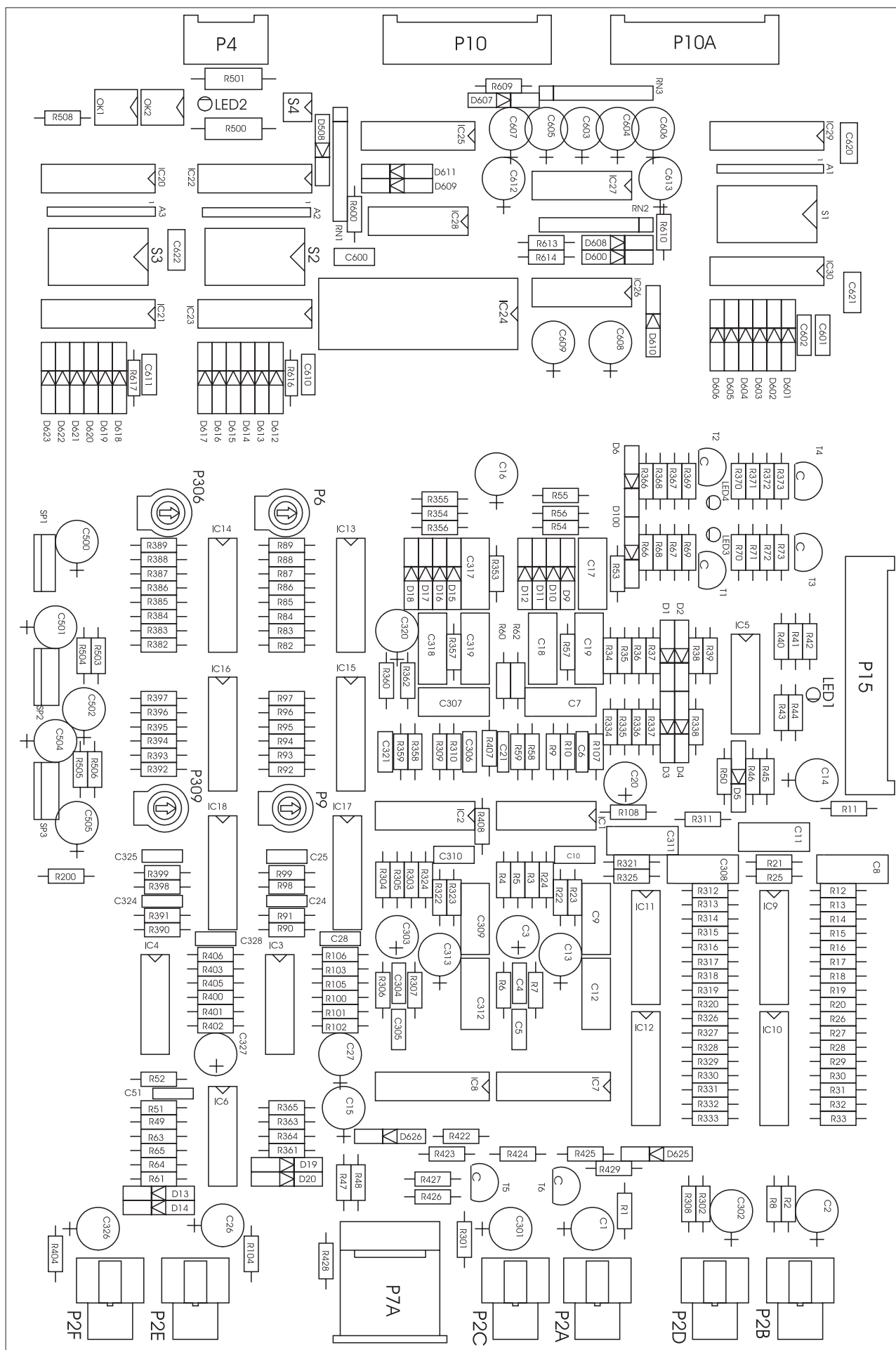
Fig. 23 - Vorverstärker vollst. / Pre-amp compl. / Préamplificateur compl.
