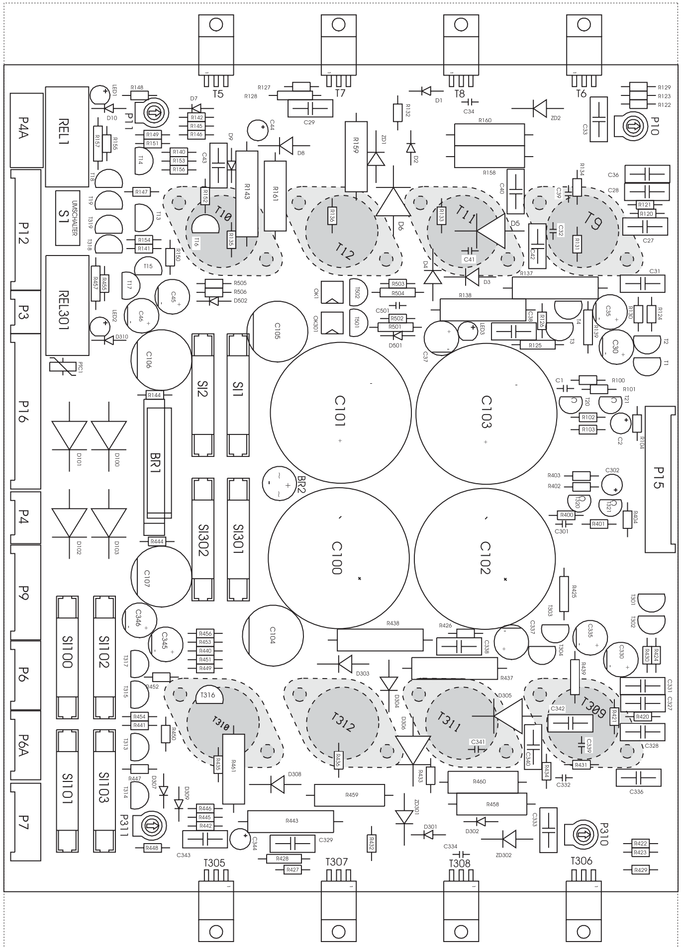
Fig. 22 - Bestückungsplan Endstufe F91 / Board layout power amplifier F91 / Tableau du tracé de puissance de l'amplificateur F91
