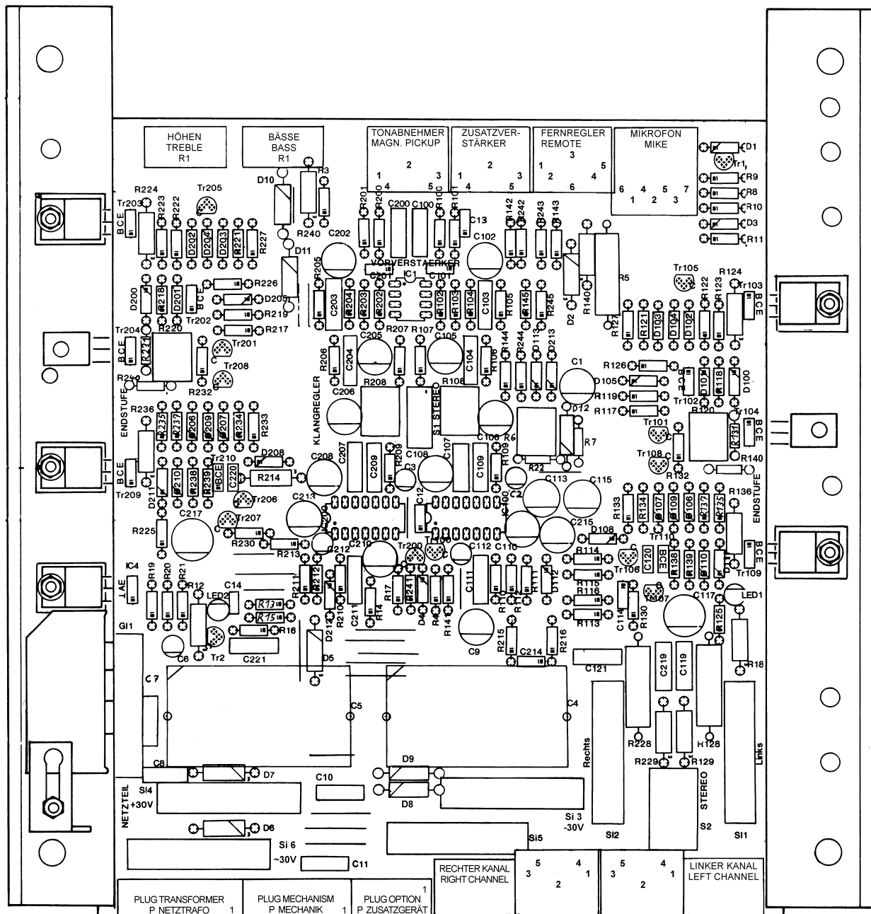
Fig. 20 - Verstärker I84, gedr. Schaltung / Amplifier I84 P.C.B. / Amplificateur I84, Circuit impr.
