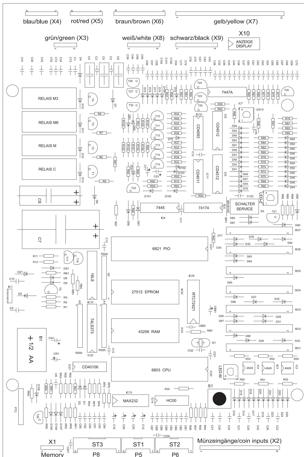
Fig. 25 - Gedr. Schaltung SCC-Steuerung / P.C.B. SCC unit / Circ. impr. unité SCC
