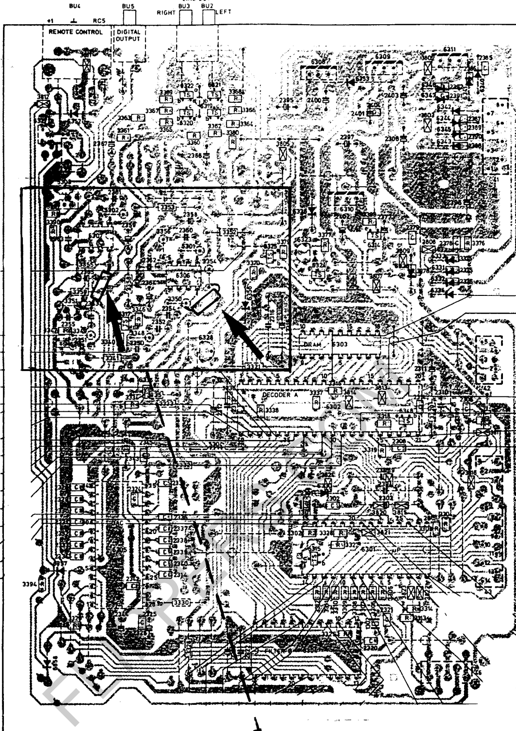
Leiterbahnunterseite Circuit board back side
